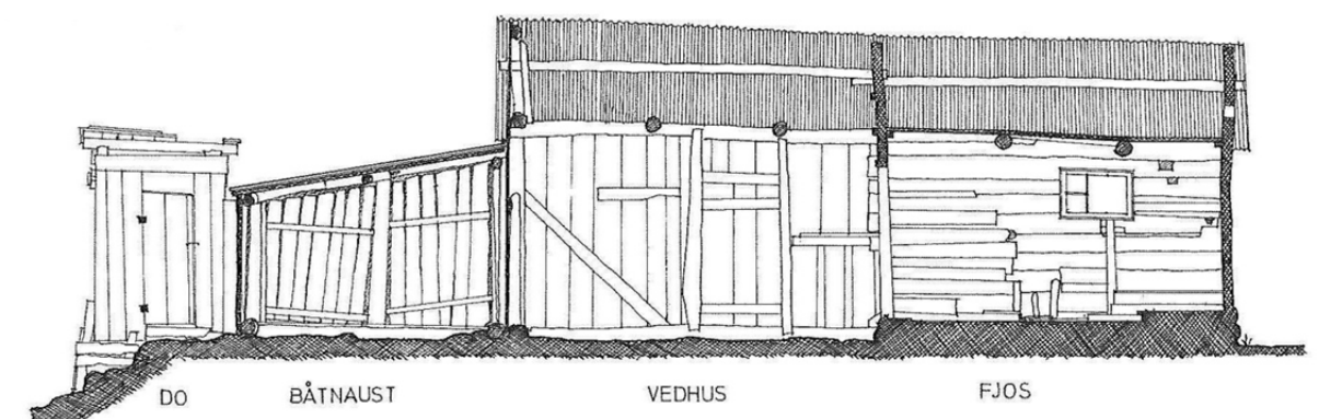
Snitt gjennom uthusbygning, studentoppmåling Gamle Lærdalsøyri
